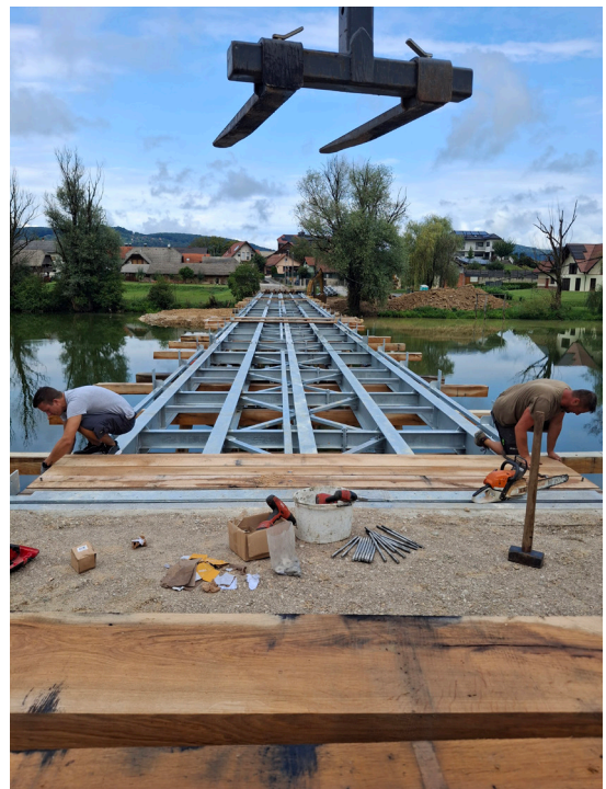
Slika 2: Most med postavljanjem kovinske konstrukcije vozišča (Foto: Judita Podgornik Zaletelj, 2025)
