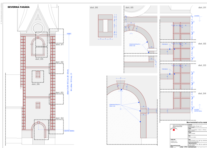
Slika 3: Arhitekturni posnetek severne fasade in detajlov poslikav registrirane kulturne dediščine Štefan pri Trebnjem – Cerkev sv. Štefana (Izdelal: Damjan Popelar, 2025)
