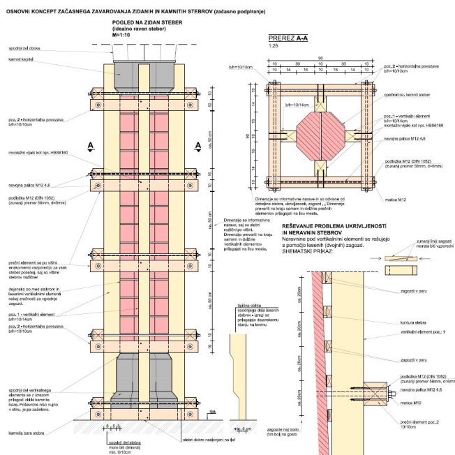
Slika 3: Načrt začasne stabilizacije slopov na podlagi predloga Pavla Pučnika, dipl. inž. gradb., Zdenka Vranješa, univ. dipl. inž. gradb., in Iztoka Leskovarja, univ. dipl. inž. gradb. (Avtorja: Zdenko Vranješ, u.d.i.g., in Pavel Pučnik, d.i.g., 2025)
