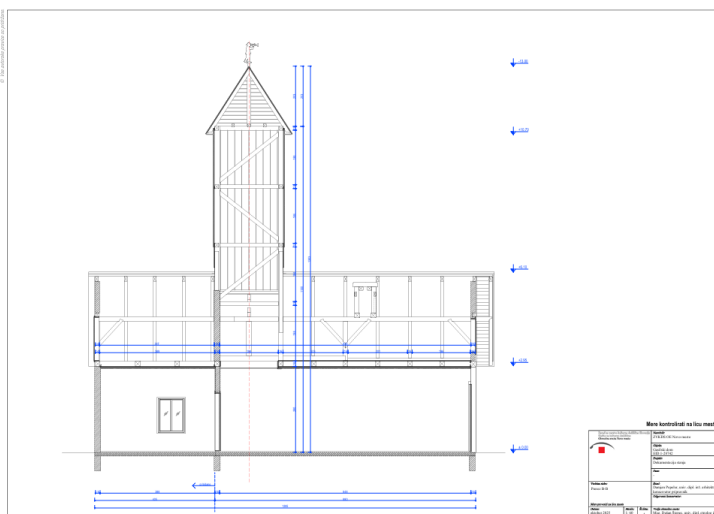
Slika 2: Prerez B-B registrirane kulturne dediščine Gradac – Gasilski dom (Izdelal: Damjan Popelar, 2025)
