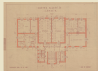
Tloris pritličja in nadstropja za mladinski dom, 1928 (arh. FAM)
