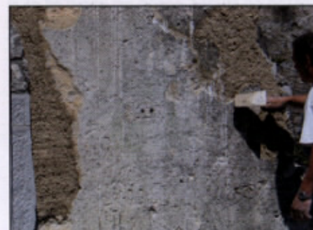
Pripravljene vzorce ometa (zgoraj) in zapolnjevanje praznih mest, Štanjel (spodaj)
