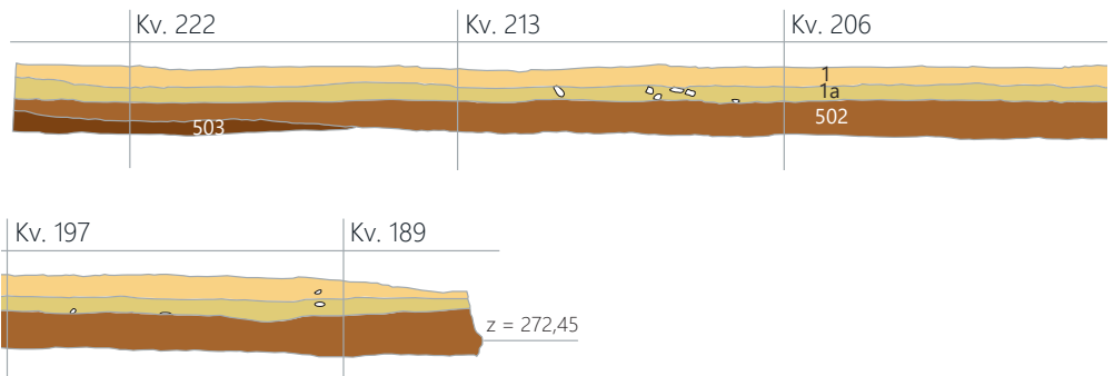
21 Presek 11. Merilo 1 : 100.
